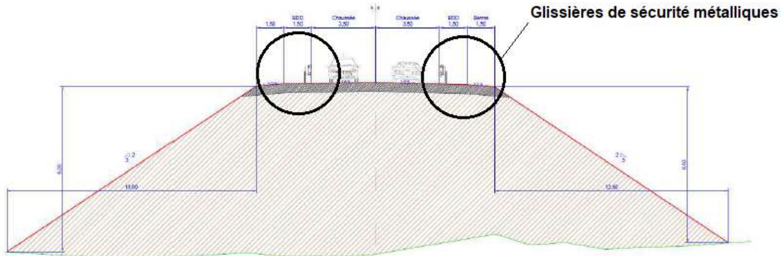
Figure 15 : Coupe A21
