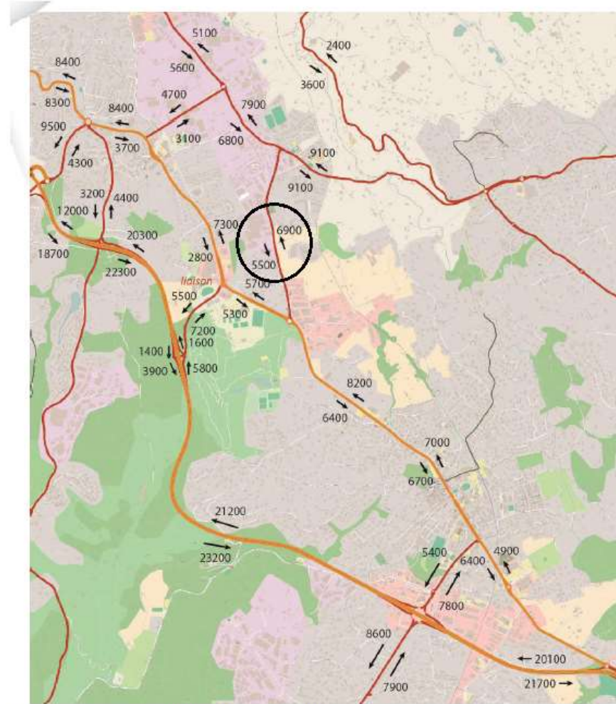
Figure 140 : Horizon 2020 – TMJA – Scénario avec le projet de liaison
