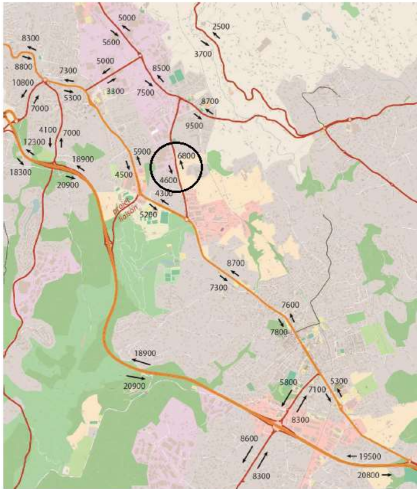
Figure 139 : Scénario de référence à l'horizon 2020 – TMJA – Scénario sans projet de liaison
