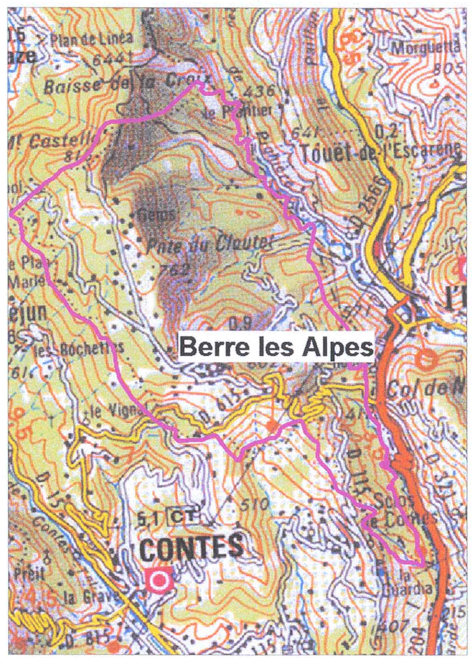
Carte des Aléas Crues Torrentielles
